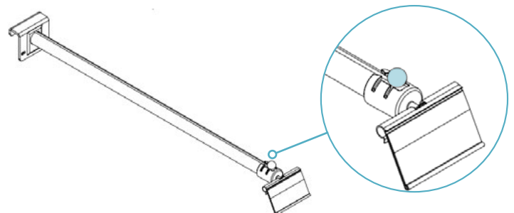
Terminación de tubo en esfera Spherical tube termination
